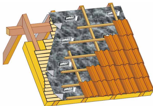
Schéma položení fólie GUTTAFOL DO 135S
