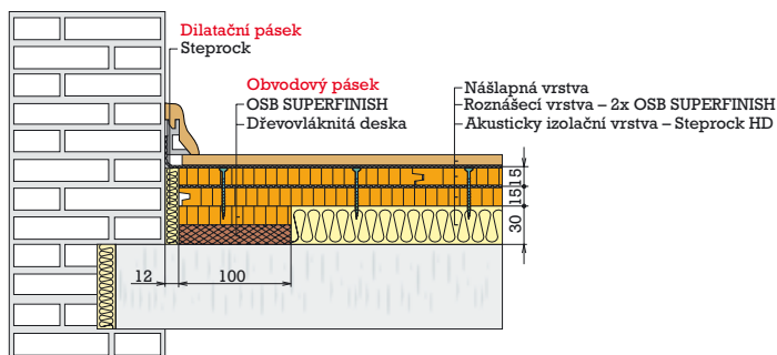
Skladba podlahy AKUFLOOR® na betonovém stropu (obr. 20)
