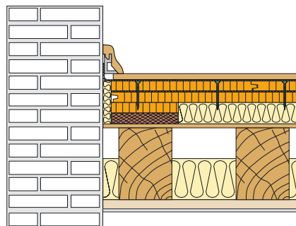
Skladba podlahy AKUFLOOR® na trémovém stropu (obr. 21)
