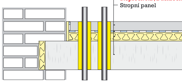
Správný prostup potrubí stropem (obr. 9)
